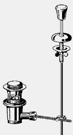
Сифон - За керамичен умивалник с преливник - Хромиран месинг
