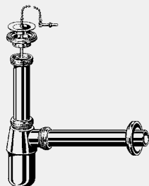
Сифон тип бутилка - Хромиран месинг Компоненти Декоративна розетка Ø 50 мм, универсален клапан от неръждаема стомана, тапа за клапан с верига Модел 5753.906
