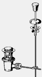
Сифон - За керамичен умивалник с преливник - Облицовка от хромиран месинг, пластмасово тяло на клапана
