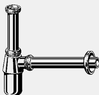
Сифон тип бутилка - Хромиран месинг Компоненти Декоративна розетка Ø 50 мм Модел 5753.904
