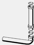
Канализационно коляно 90° - Пластмаса Компоненти Отходна тръба Модел 5632.2
