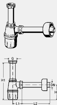
Sifon - plastika Oprema Posuda Ø 50 mm Model 5725
