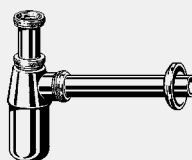
Sifon - hromirani mesing Oprema Posuda Ø 60 mm, rozetna, prilagodljiva cev 95 mm, odvodna cev 200 mm sa kontrolom kvaliteta prema DIN EN 274 Model 5763
