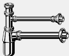
Sifon - hromirani mesing Oprema Posuda Ø 50 mm, prilagodljiva navojna spojnica, priključak za prodirnu vodu, podesiva cev 160 mm, odvodna cev 250 mm sa kontrolom kvaliteta prema DIN EN 274 Model 5753.02
