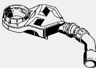
Advantix-Sifon (model za saniranje) - za sledeće komponente ili namene: prepravljanje Advantix-ugaonih odvoda na visinu ugradnje 66 mm - nije odgovarajući za sledeće komponente ili namene: Advantix-ugaoni odvod model 4973.81 - odgovara za sledeće komponente ili namene: Advantix-ugaoni odvod model 4972.80, 4972.81, 4972.82, 4972.83
